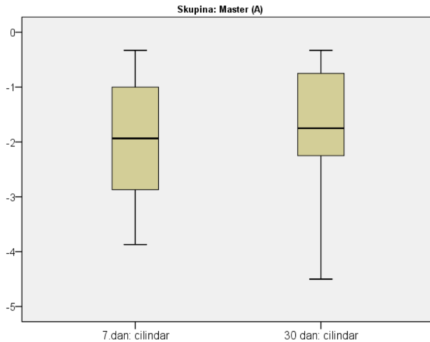
Slika 12 Razlike između 7. i 30. dana u cilindrima u skupini Master
