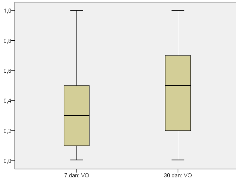
Slika 6. Razlike između 7. i 30. dana u VO na cjelokupnom uzorku
