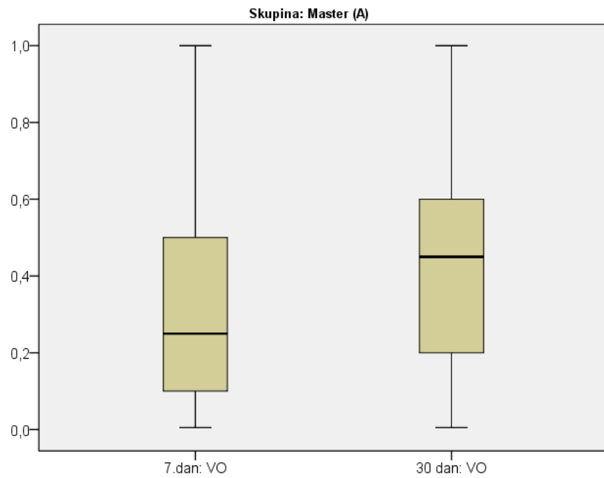
Slika 11 Razlike između 7. i 30. dana u VO u skupini Master
