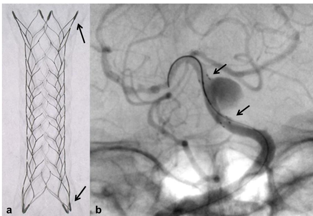
Slika 6. Nitinolska samošireća intrakranijska potpornica. a) fotografija jedne od korištenih potpornica, b) angiografsko snimanje nakon postavljanja potpornice preko vrata aneurizme na bazilarnoj arteriji (strelice pokazuju njene krajeve).
